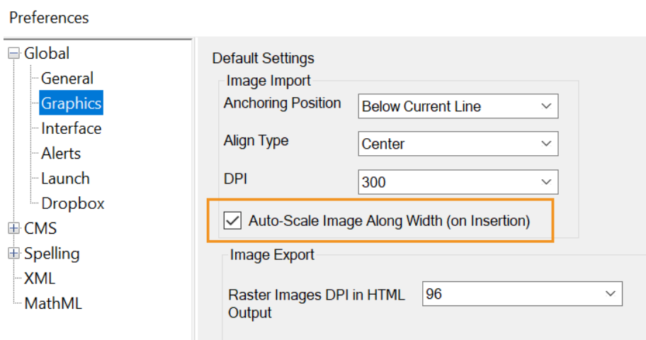
Figure 1: 環境設定ダイアログの画像自動拡大 / 縮小オプション
