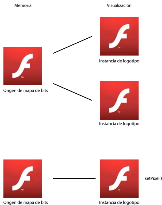
Resultado en memoria de la modificación de un mapa de bits
