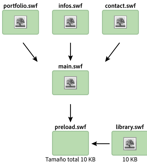
Uso de una biblioteca compartida en tiempo de ejecución.
