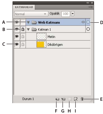
A. Katmanı Genişlet/Daralt B. Katmanı Kilit/Kilidini Aç C. Katmanı Göster/Gizle D. Etkin Katman E. Katmanı Sil F. Yeni/Çoğaltılmış Katman G. Yeni Alt Katman H. Maske Ekle I. Yeni Bitmap Görüntüsü
