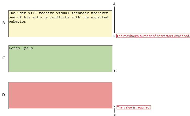
A. Räknare för antal kvarstående tecken B. widgeten Textområde i fokus, läget högsta antal tecken C. widgeten Textområde i fokus, giltigt läge D. widgeten Textområde, obligatoriskt läge E. Räknare för antalet inskrivna tecken
