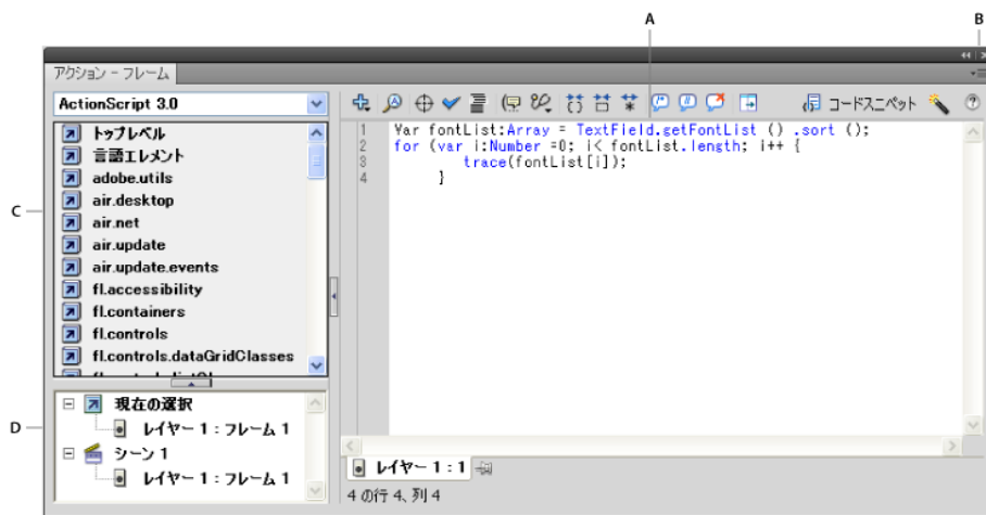
A. スクリプトペイン B. パネルメニュー D. スクリプトナビゲーター
