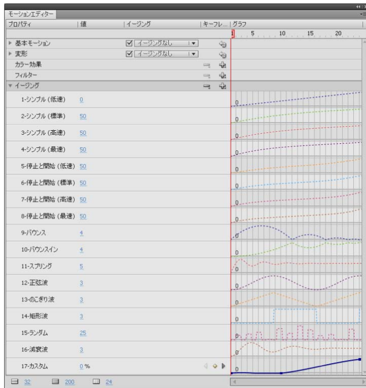
Flash に含まれるイーasing曲線の形
