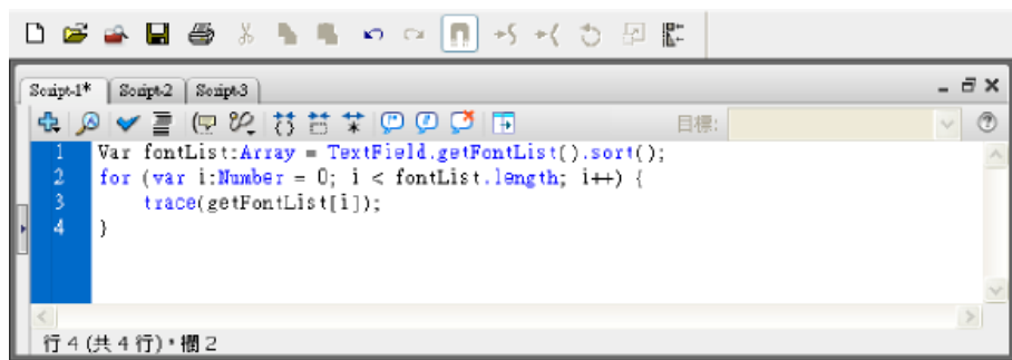
スクリプトウィンドウ
