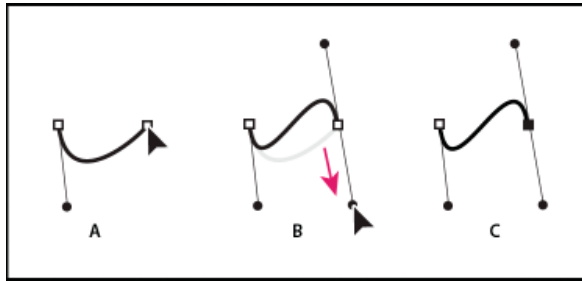
S 字曲線の描画
