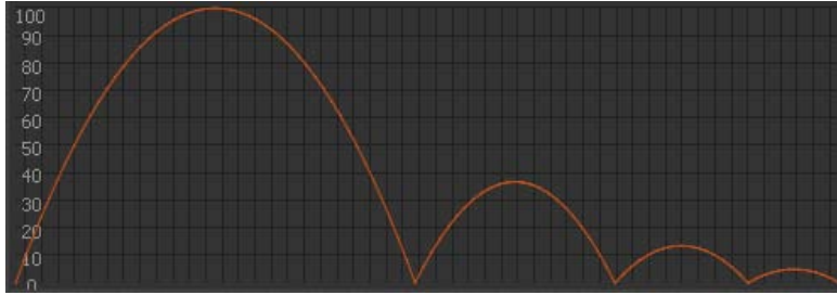
バウンスプリセットイージングで描画された曲線
