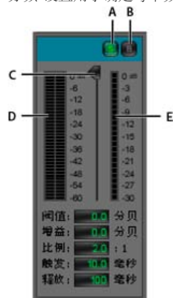
多频段压缩器中特定于频段的控件
