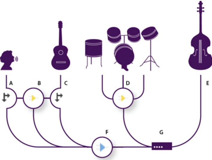
轨道音频路由示例
