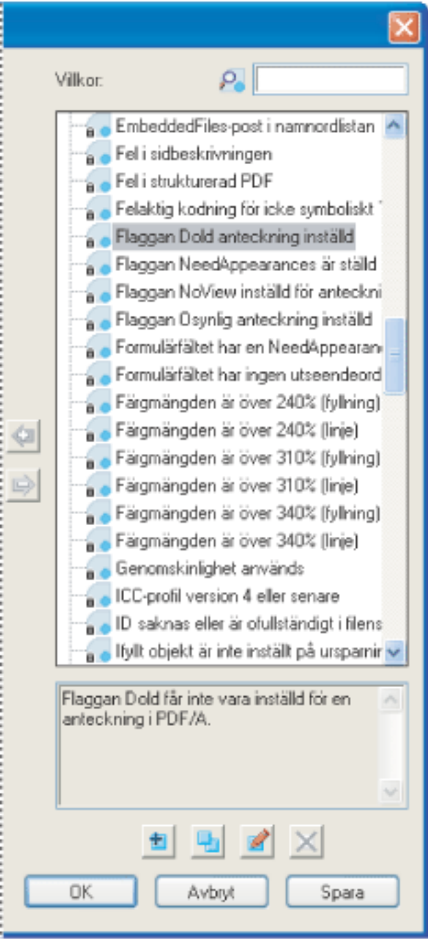
Kolumnen Villkor i dialogrutan Redigera profiler
