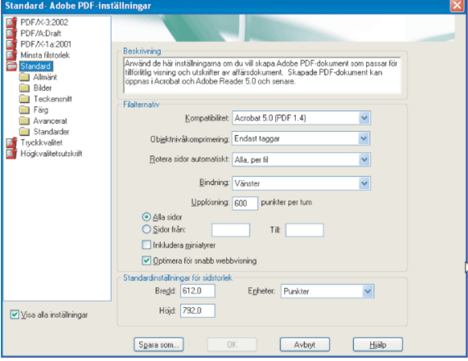
Dialogrutan Adobe PDF-inställningar med panelen Allmänt
