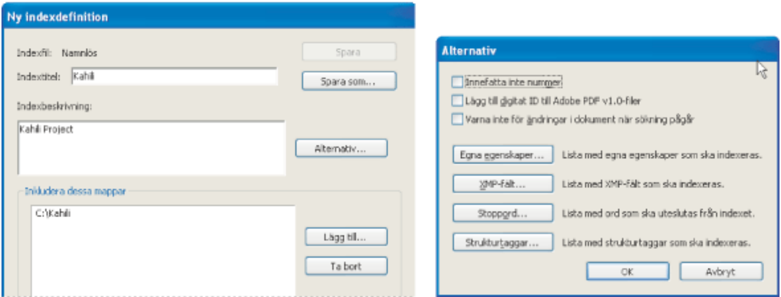
Indexdefinitioner (vänster), indexalternativ (höger)
