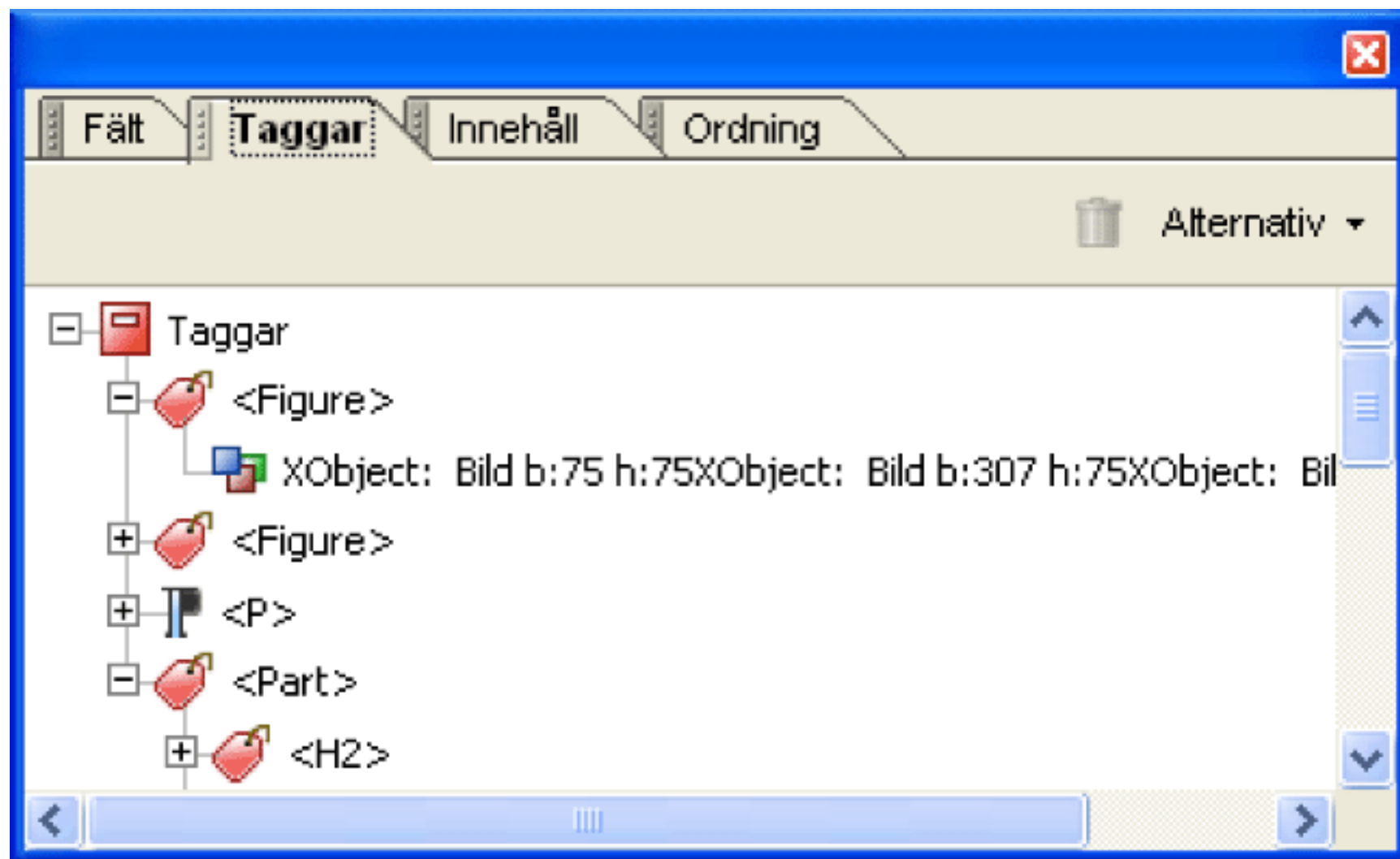
Det logiska strukturträdet på fliken Taggar
