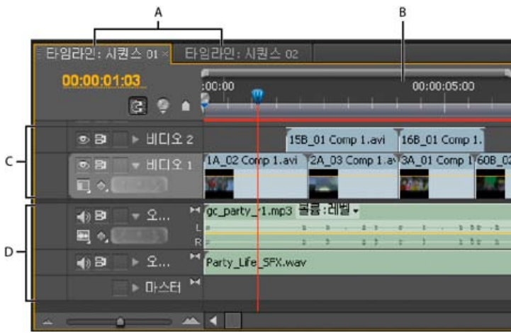
타임라인 패널
