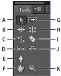
도구 상자
