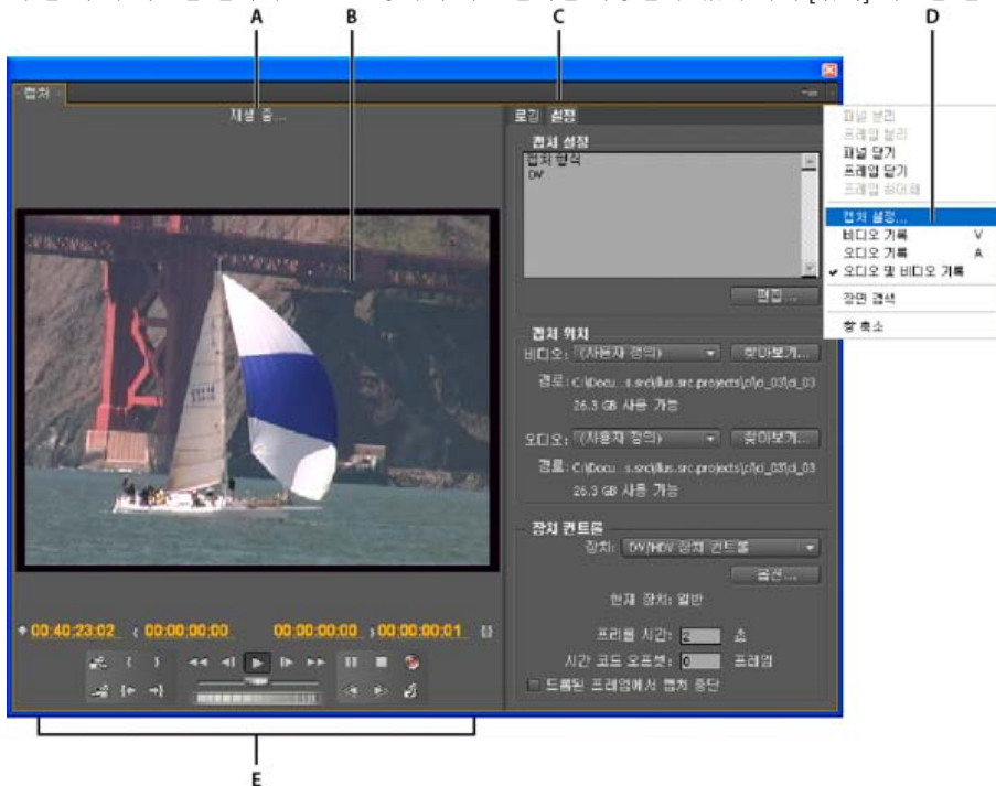
캡처 패널
