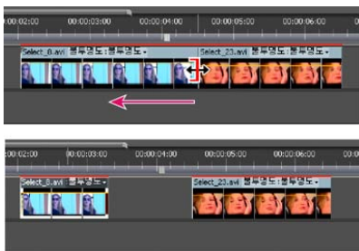
클립 트리밍
