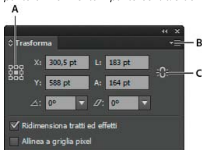
Pannello Trasforma
