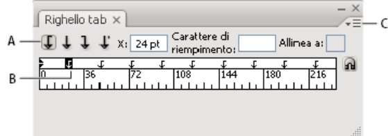
Tabulazioni ripetute
